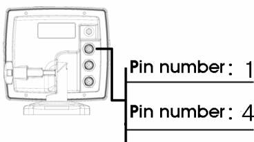
Input (1) NMEA 0183
