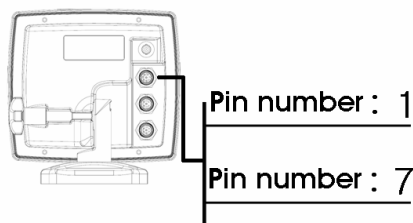
Input (2) NMEA 0183
