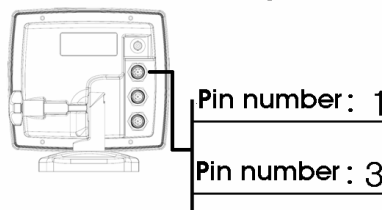
Output (1) NMEA 0183
